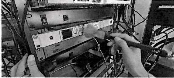
Remoción de polvo a la electrónica de la micro onda
